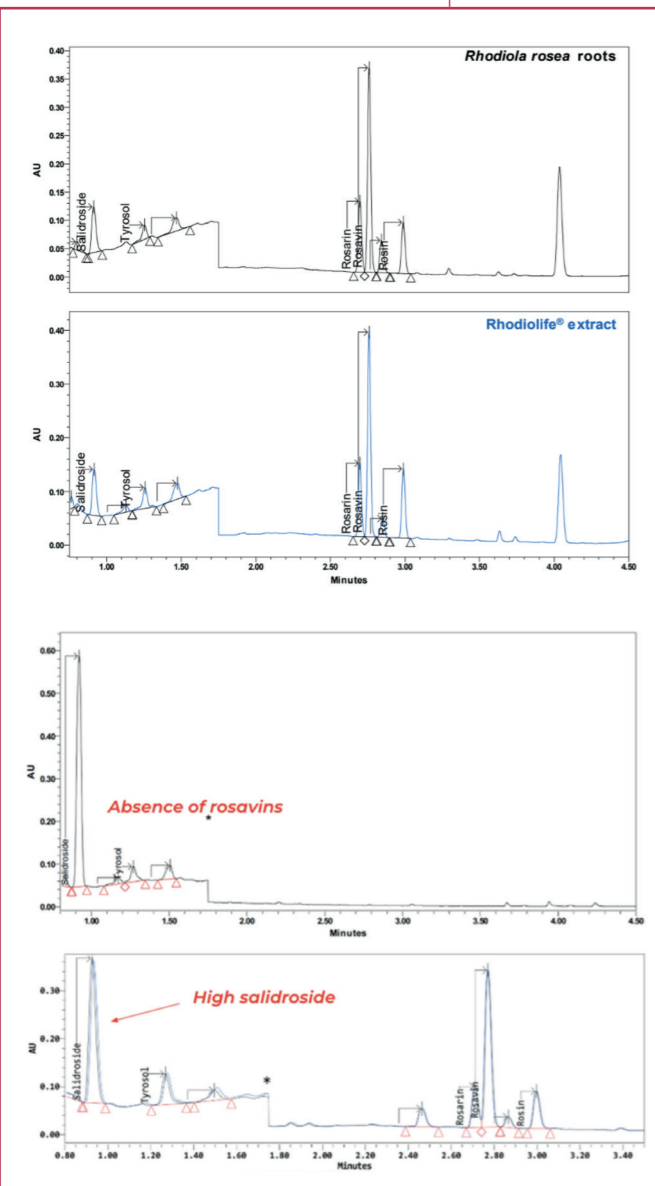
Spettri molecolari di estratti di Rhodiola rosea a confronto: estratto pianta nativa, Rhodiolife® ed estratti adulterati
